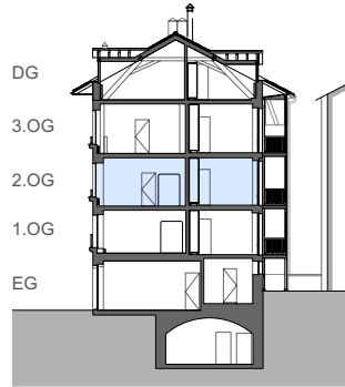
Schnitt
