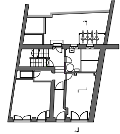
Eingangsgeschoss
